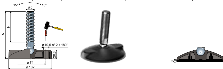
Размеры штока в мм / Medidas del vástago en mm
